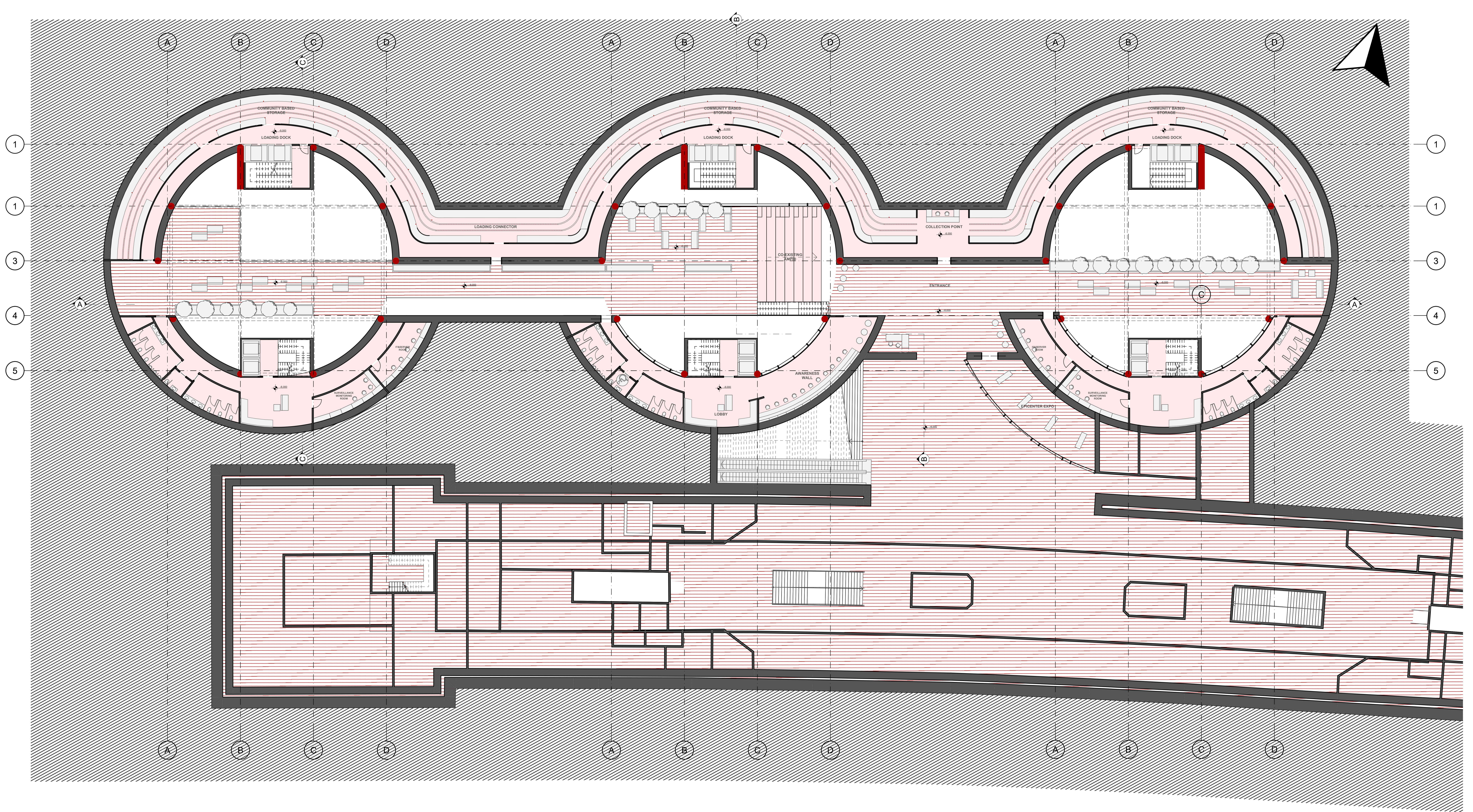
PLAN (-6.00 m) SCALE: 1/200
