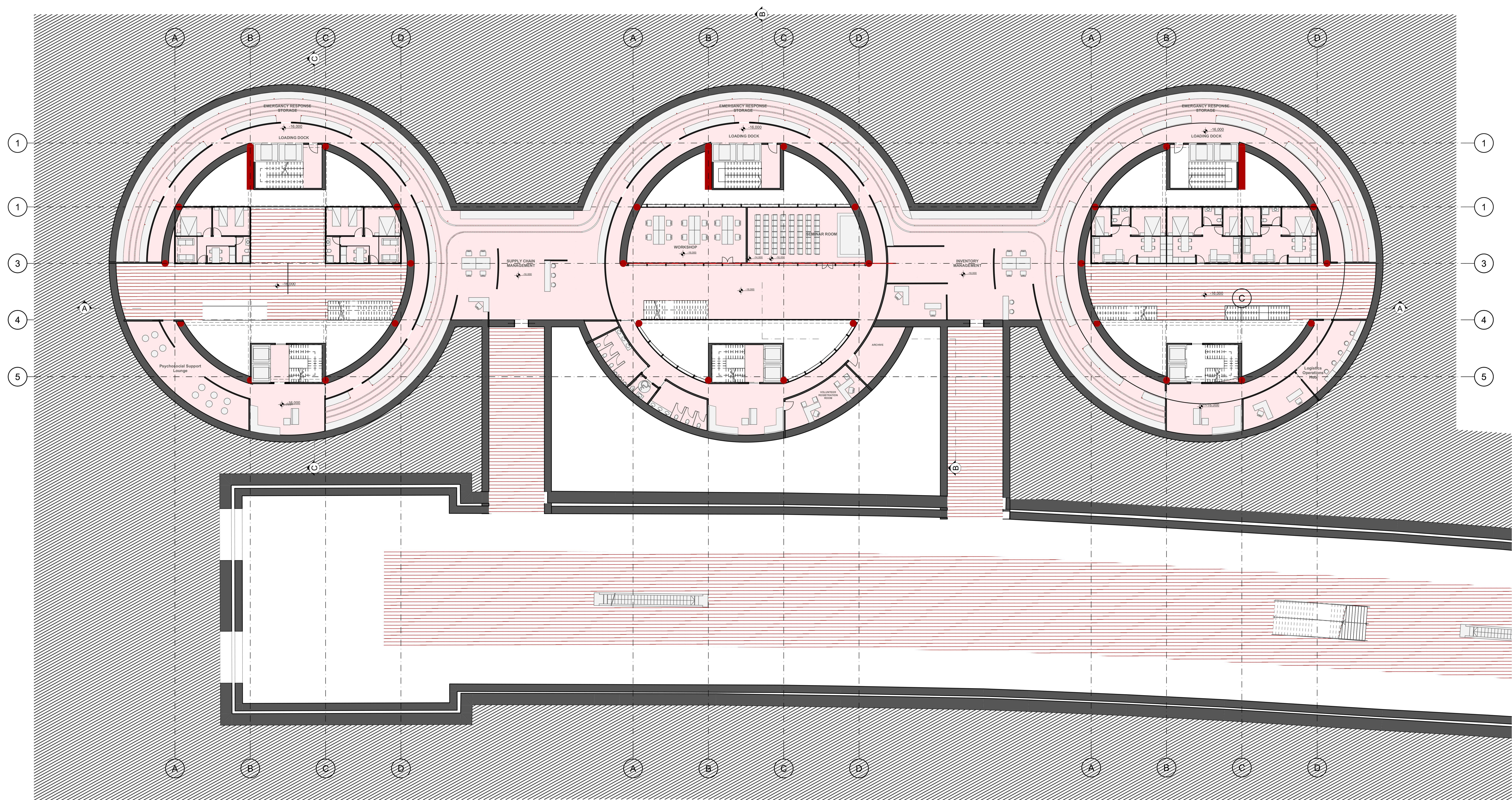
PLAN (-14.00 m) SCALE: 1/200
