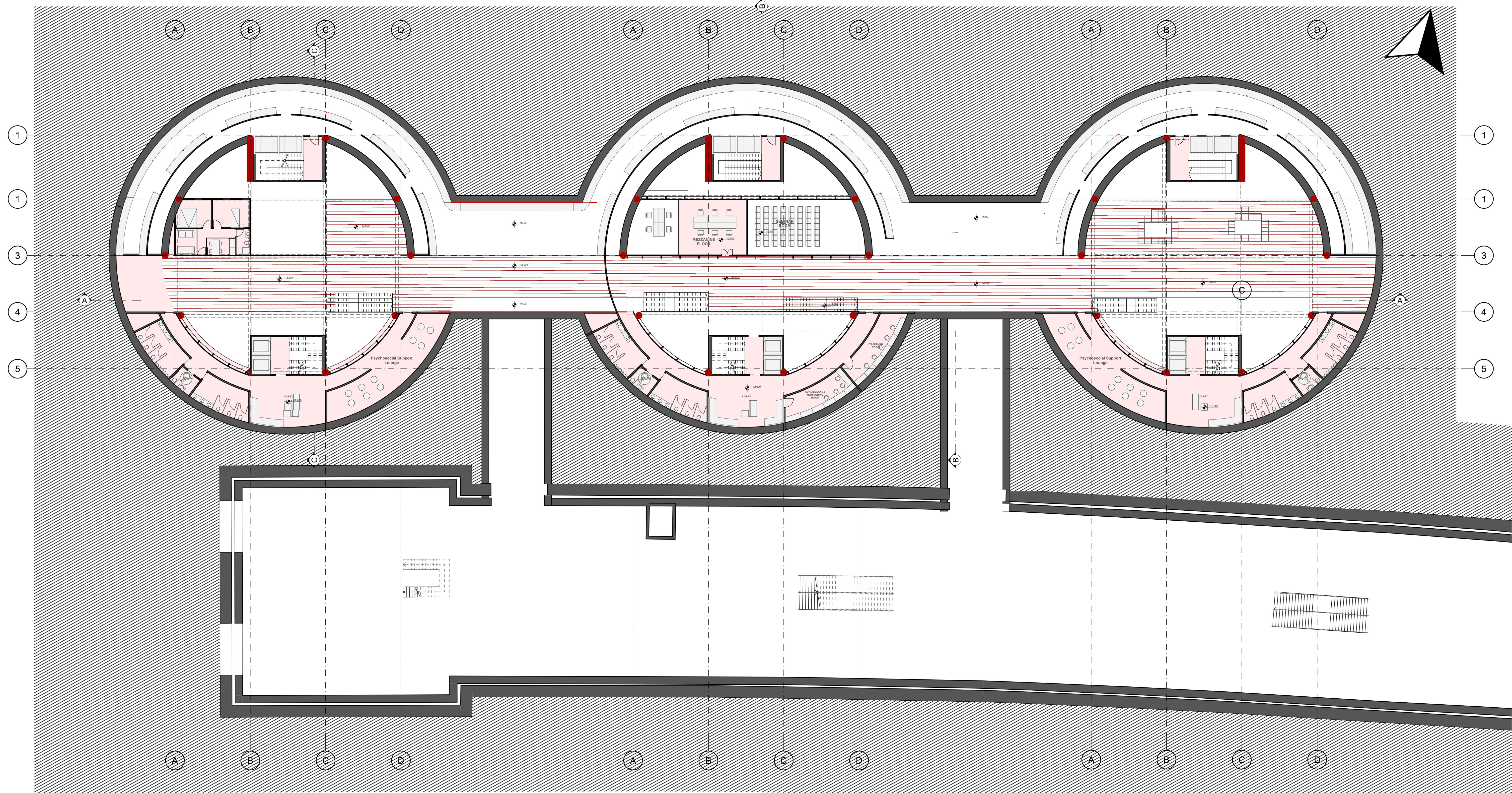
PLAN (-10.00 m) SCALE: 1/200
