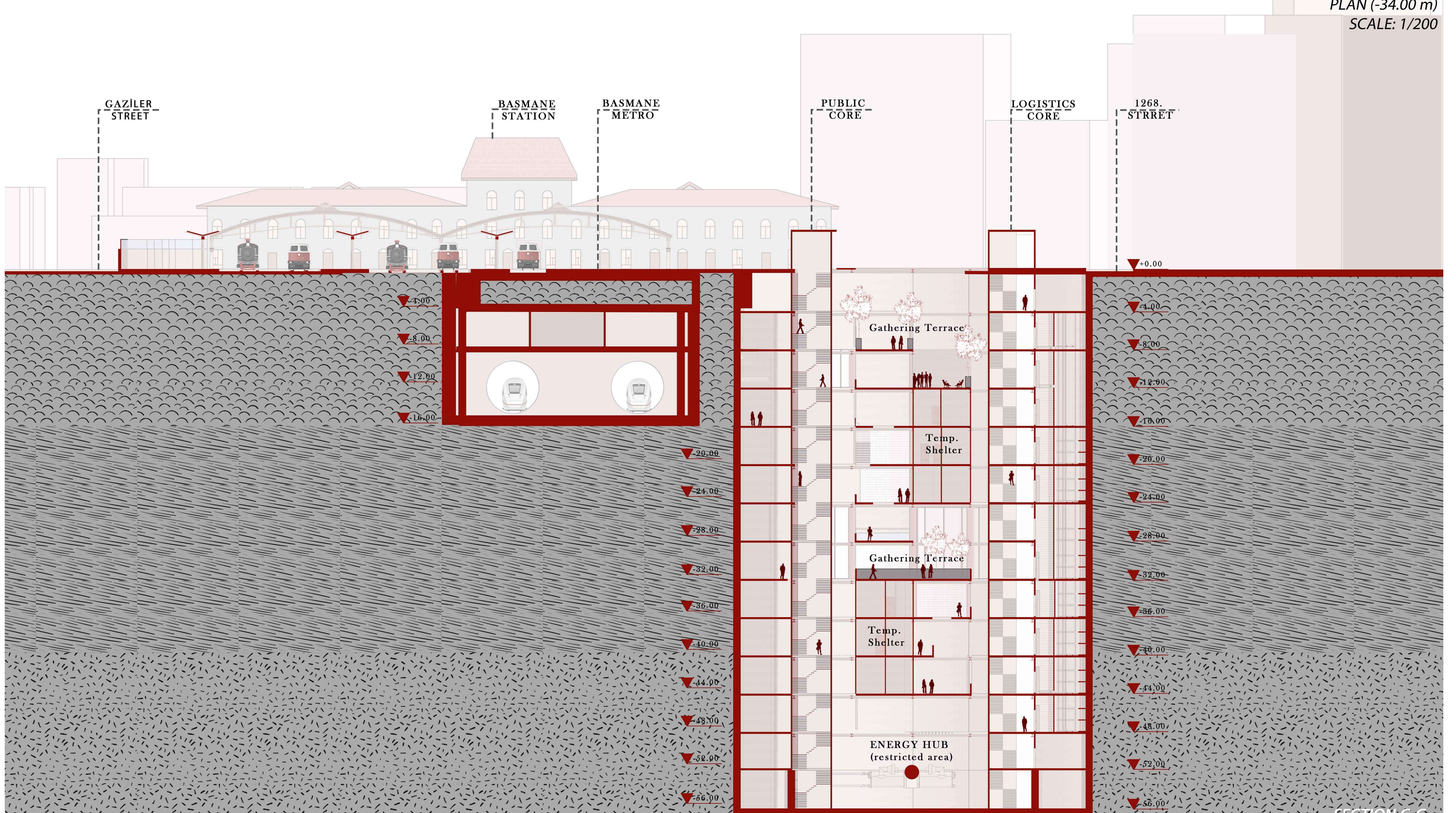
SECTION C-C SCALE: 1/200
