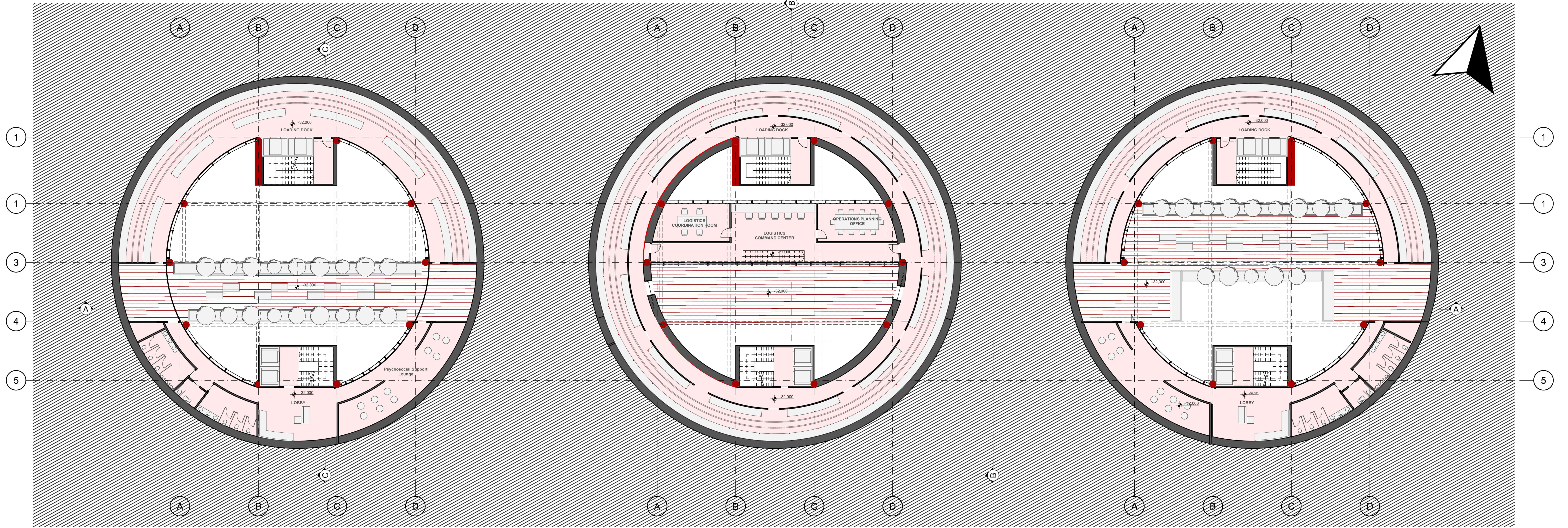
PLAN (-30.00 m) SCALE: 1/200
