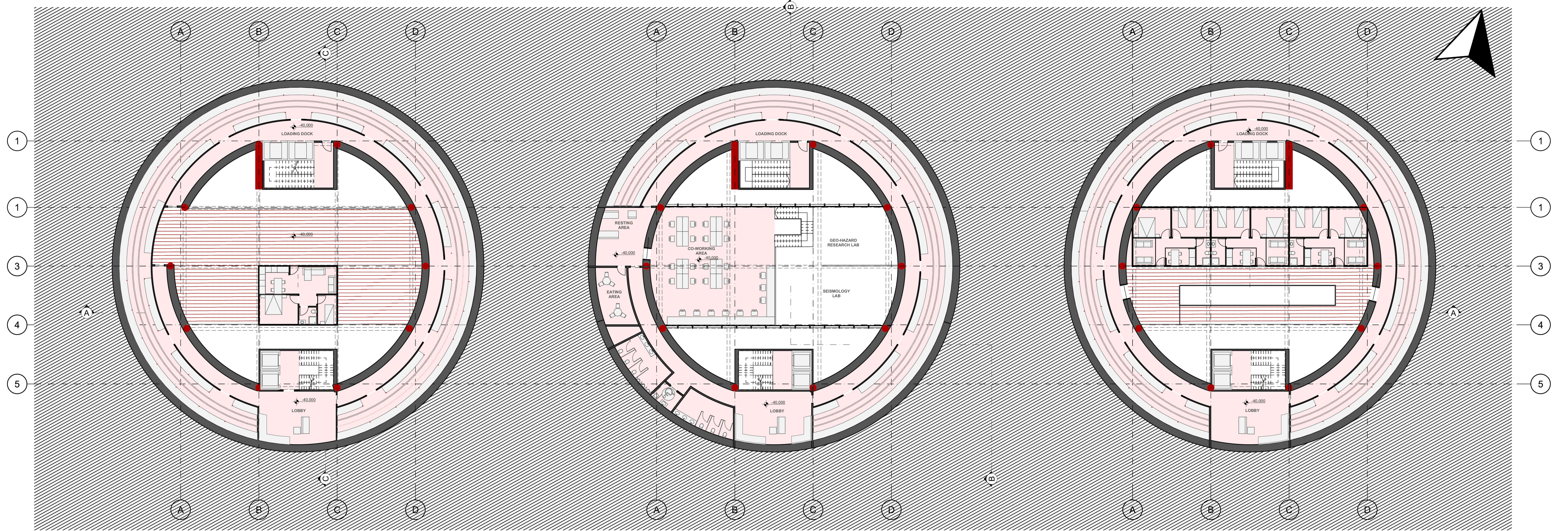
PLAN (-38.00 m) SCALE: 1/200
