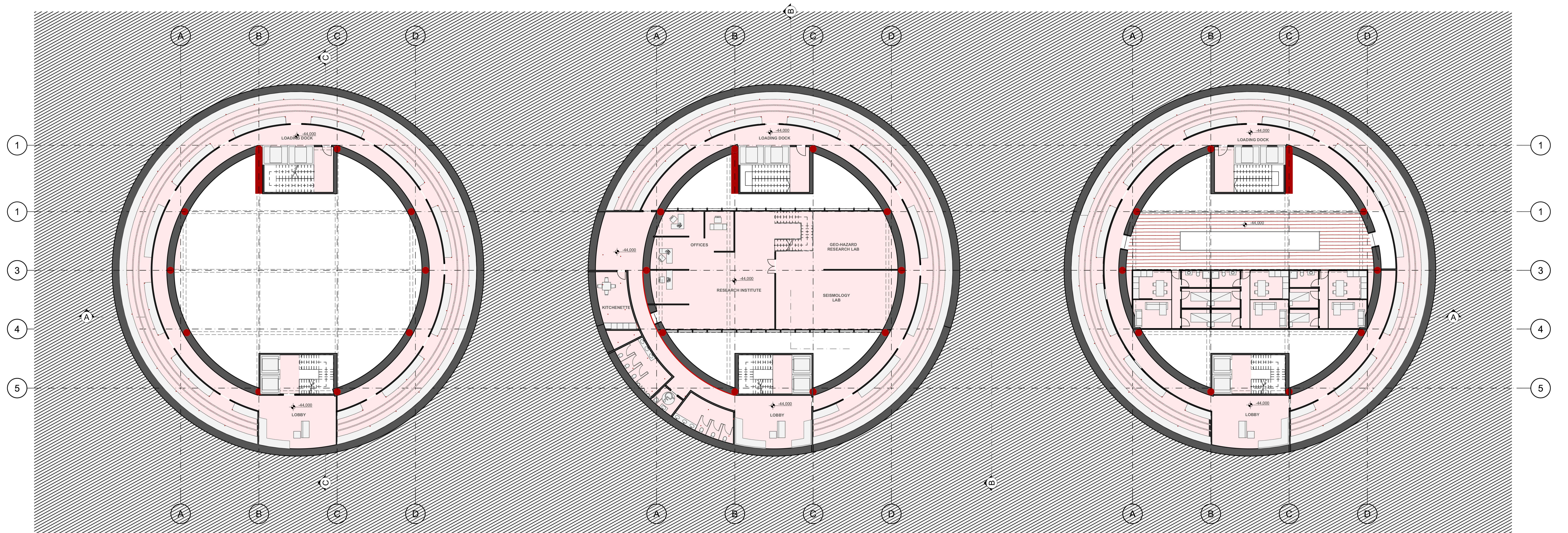
PLAN (-42.00 m) SCALE: 1/200
